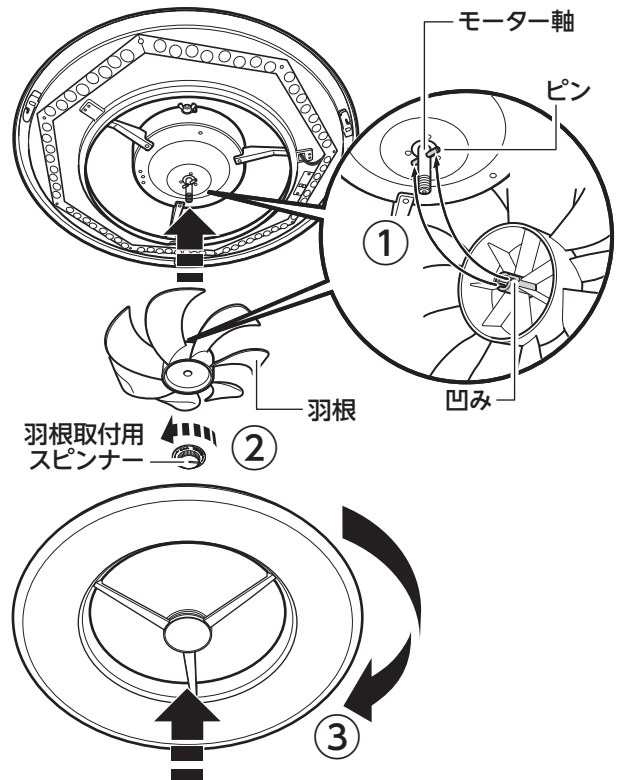
羽根の取り付けかた
